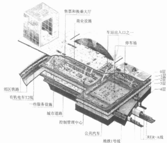
图 3 巴黎拉德芳斯枢纽站剖面图 [4]
