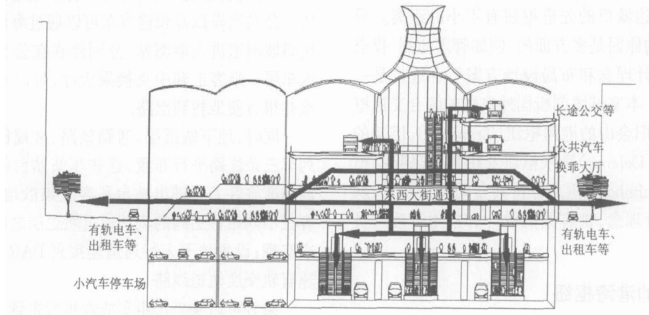
图 2 旧金山港湾枢纽立面布局 [3]
