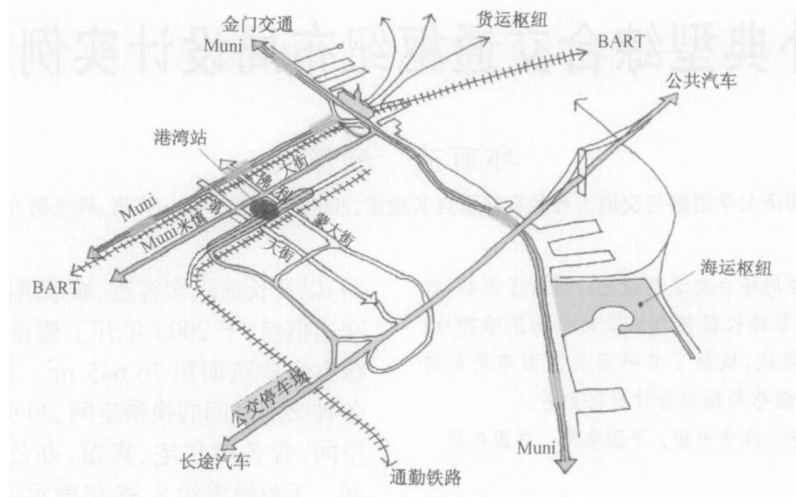
图 1 旧金山港湾枢纽平面布局 [3]
