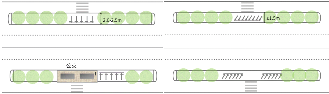
图 9.3.1 自行车停车设施结合绿化带、设施带设置示意
