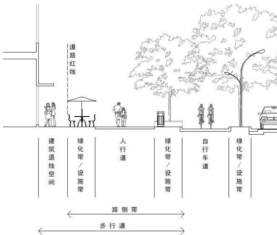
图 5.1.2 - 1 步行道和自行车道横断面示意
