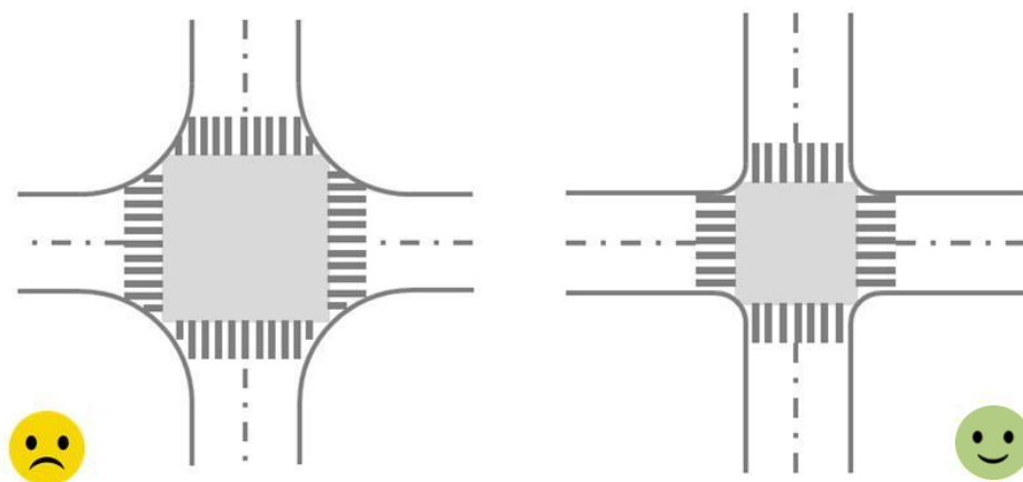
图 5.5.1 交叉口转角路缘石小转弯半径反例与正例
