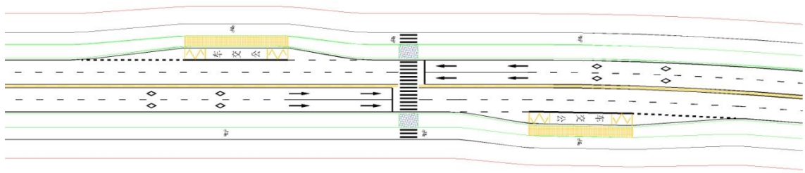
图 11.2.3 行人过街设施与公交站结合设置平面布局示意
