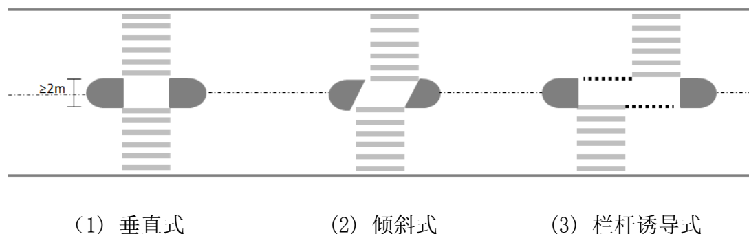
图 5.4.8 安全岛类型示意
