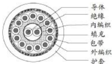
图 A.2 16 芯线缆截面图
